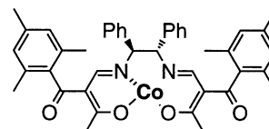
Fig. 1. ( S )-MPAC ( 1a ).
